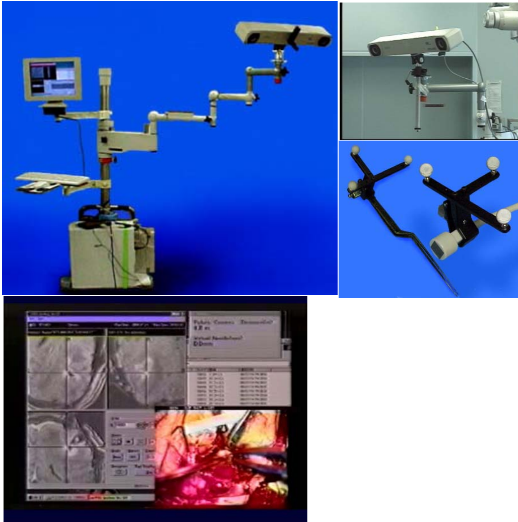
図 2.5.2-1 手術用ナビゲーション装置(東京女子医科大学) 3)
